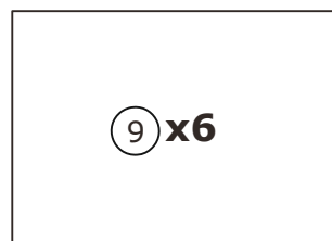
298x278x2 mm
